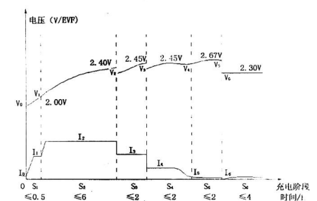
1. 充电曲线示意图:
